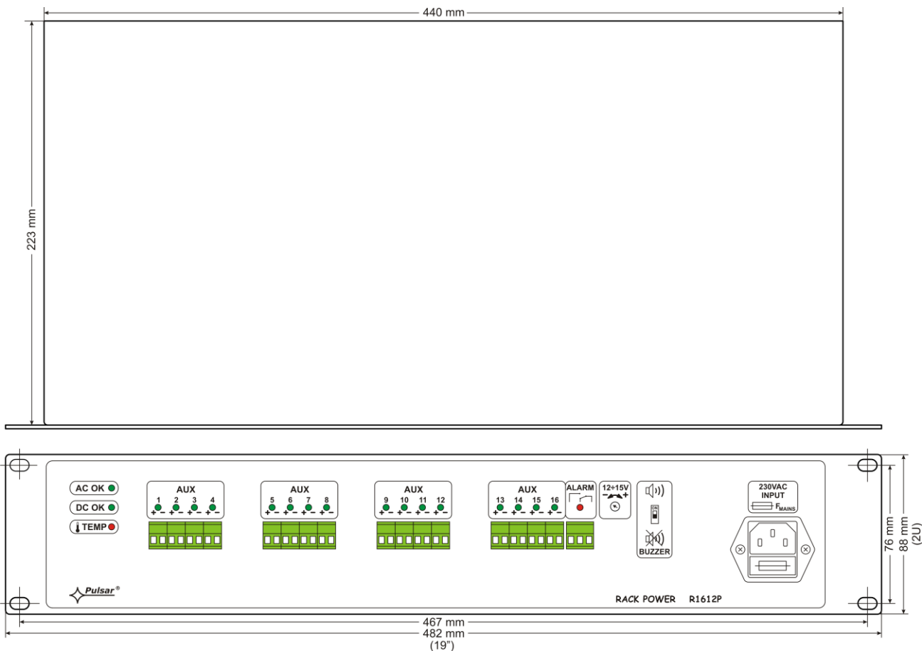
Rys.3. Widok zasilacza.
