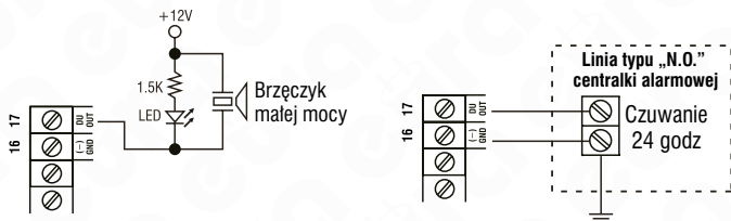
Rys. 16. Wykorzystanie wyjścia „DURESS” (patrz opis w rozdz.5.6.6).
