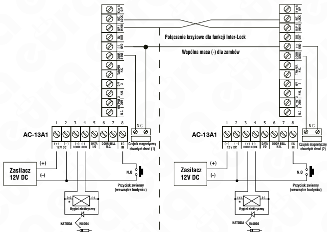
Rys. 9. Wzajemne połączenie 2 zamków AC-13A1 w systemie „Inter-Lock”
