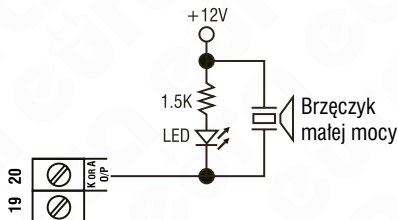
Rys. 13. Podłączenie wyjścia alarmowego zamka do prostego brzęczka i diody LED.
