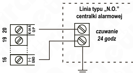
Rys. 12. Podłączenie wyjścia alarmowego zamka do zewnętrznej centrali alarmowej
