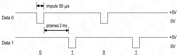
Rys. 6. Sygnały elektryczne na liniach wyjścia Wiegand
