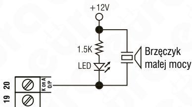
Rys. 14. Podłączenie wyjścia alarmowego prostego brzęczka i diody LED, które dźwiękiem i światłem przez 10 sekund potwierdzą wciśnięcie dowolnego klawisza na klawiaturze
