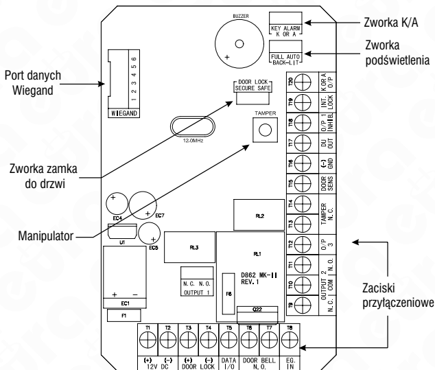
Rys. 2. Rozkład zacisków elektrycznych na płytce drukowanej zamka.
