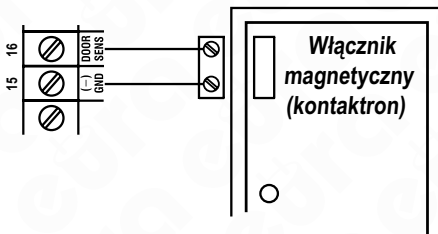
Rys. 11. Wykorzystanie wejścia z magnetycznego czujnika otwartych drzwi.
