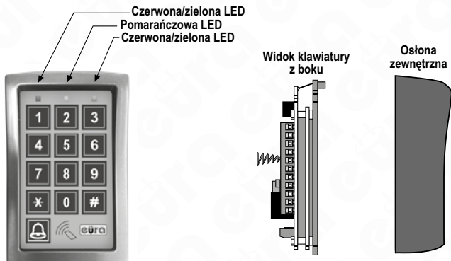
Rys.1. Budowa zamka szyfrowego AC-13A1
