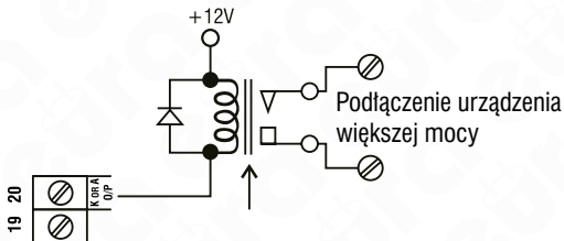
Rys. 15. Podłączenie wyjścia alarmowego do innych urządzeń, które uruchomią się na 10 sekund po wciśnięciu dowolnego klawisza
