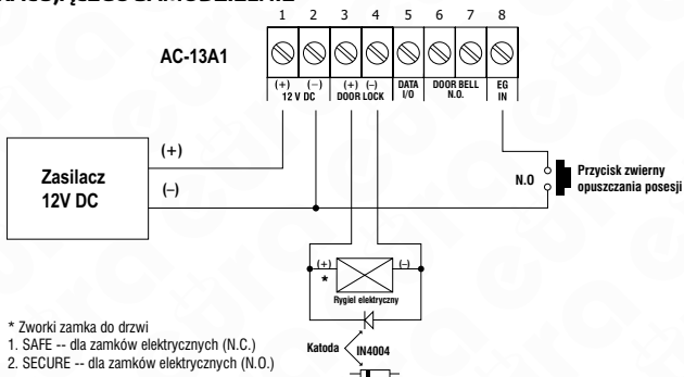
Rys. 8. Schemat podstawowy podłączenia zamka AC-13A1
