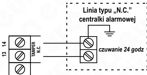
Rys. 10. Podłączenie wyjścia antysabotażowego „TAMPER N.C.” do zewnętrznego systemu alarmowego
